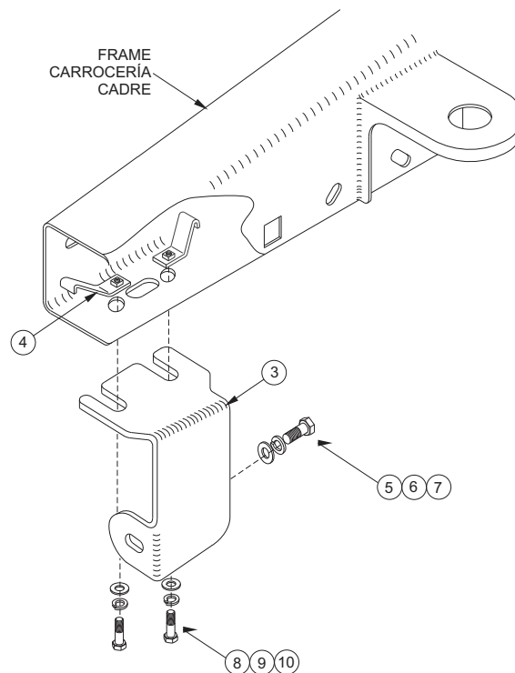
FIGURE 1 INSTALLATION VIEW OF DRIVER SIDE SHOWN, PASSENGER SIDE OPPOSITE FIGURA 1 VISTA DE LA INSTALACIÓN DEL LADO DEL CONDUCTOR OPUESTO AL LADO DEL ACOMPAÑANTE FIGURE 1 ILLUSTR: COTE CONDUCTEUR, EN FACE: COTE PASSAGER
