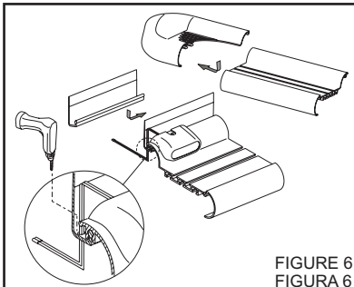
AUXILIARY LIGHT SOURCE (IF EQUIPPED) FUENTE DE LUZ AUXILIAR (SI ESTÁ INCLUIDA) SOURCE DE LUMIERE AUXILIAIRE (SI EQUIPE)
