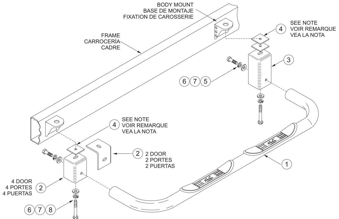
INSTALLATION VIEW OF DRIVER SIDE SHOWN, PASSENGER SIDE OPPOSITE VISTA DE LA INSTALACIÓN DEL LADO DEL CONDUCTOR OPUESTO AL LADO DEL ACOMPAÑANTE ILLUSTRÉ: COTE CONDUCTEUR, EN FACE: COTE PASSAGER
